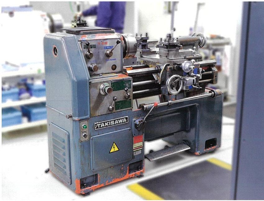
株式会社滝澤鉄工所製 小型普通精密旋盤 TSL-550
