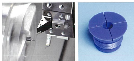
DMG 森精機株式会社製 ターニングセンタ ALX2000
